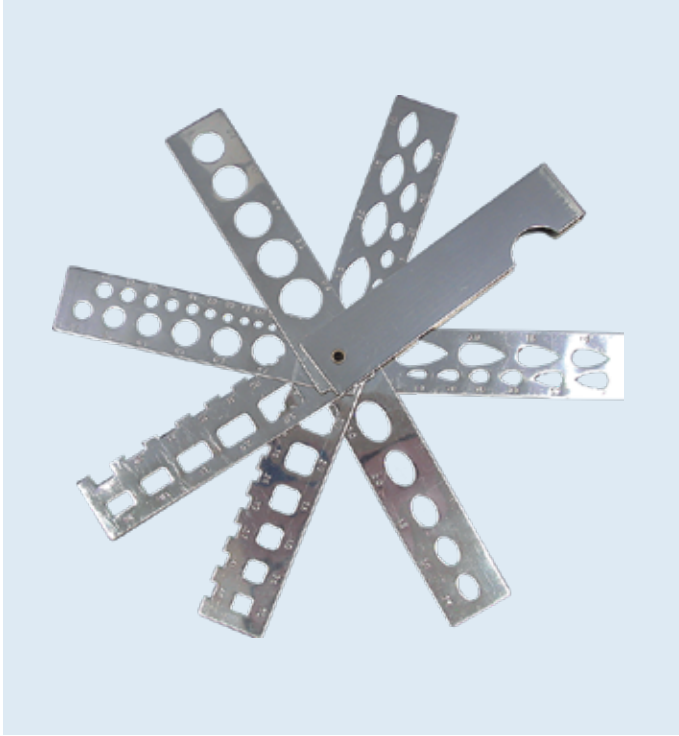
8070 Calibrador de 7 brazos para piedras redondas $258.00 + IVA
